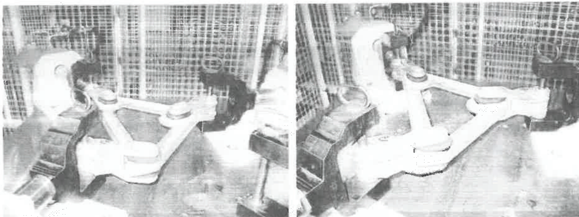
Fig. 3 – Устройство за симулация на ток на късо
